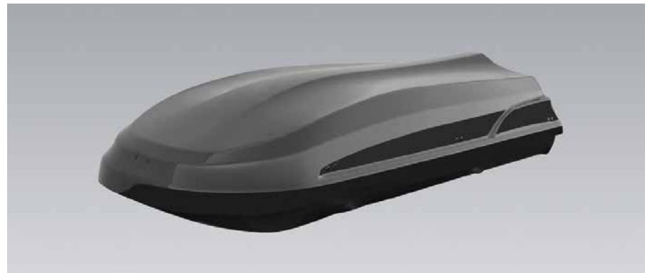
Dachbox "Adamantis". Volumen: 460 Liter, Maße: 185 x 80 x 42cm, Farbe: anthrazit, doppelseitig öffnend. 9999Z-04197
